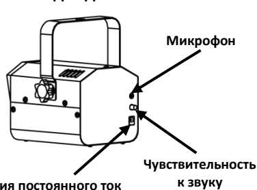
Вид задней панели
