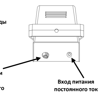
Вид задней панели
